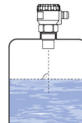
Fig.1 Instalação recomendada
